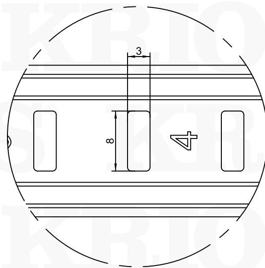
Dettaglio/Detail B
