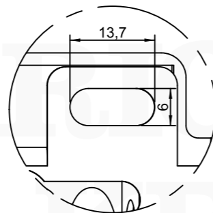
DETTAGLIO B
